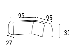
schienale "angolare" "corner" back
