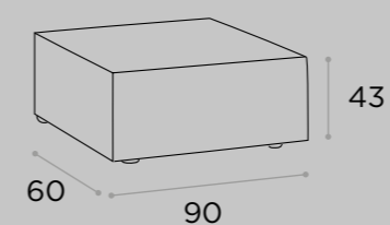
ALOE rettangolare
